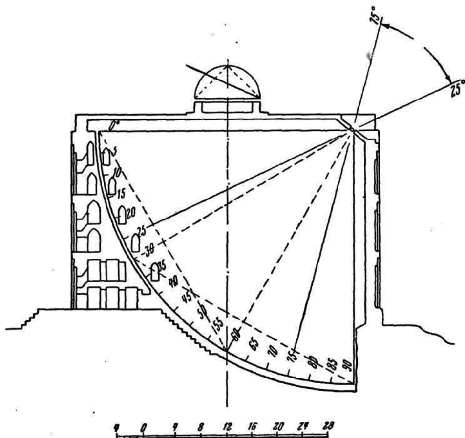
Рис. 44. Обсерватория Улугбека. Разрез север — юг.
